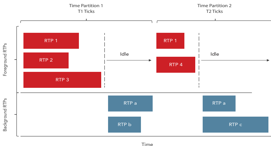
图2：VxWorks功能安全套件的前台和后台进程
