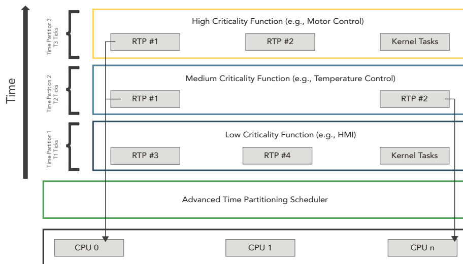
图1：示例中的VxWorks功能安全套件 时间片调度器的配置包含3个时间片和CPU对应关系（用箭头表示）
